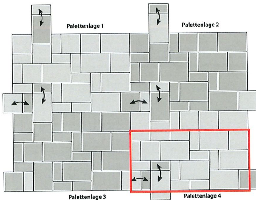
Bild 2: Verlegefläche
